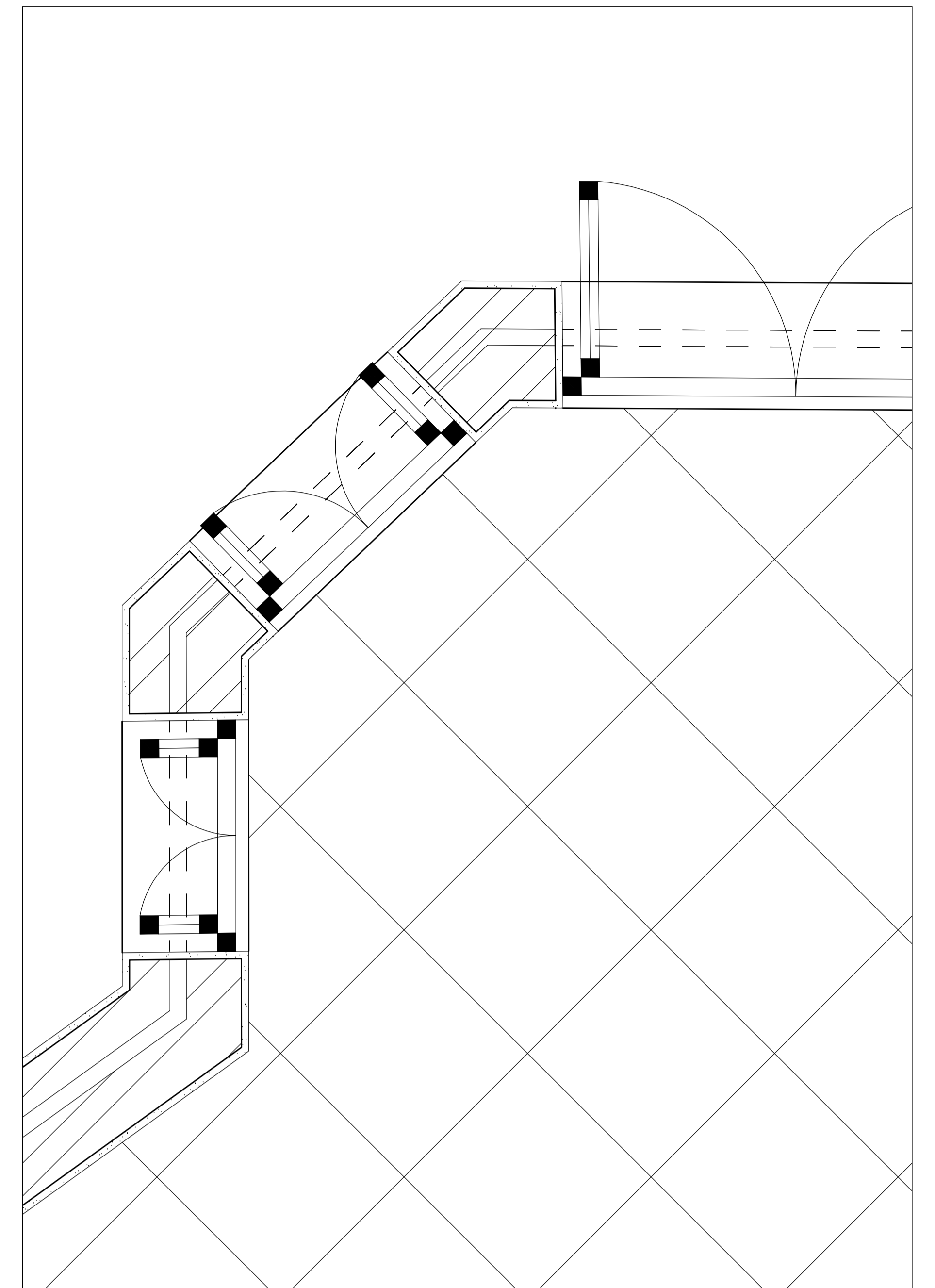
Pormenor Janelas 1/10
