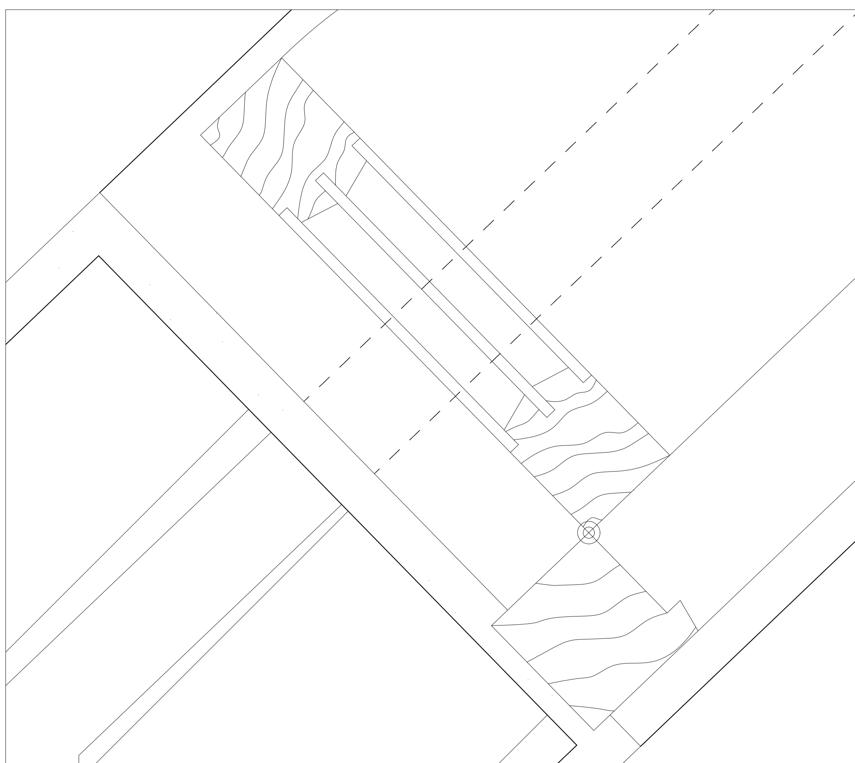
Pormenor Janelas 1/1
