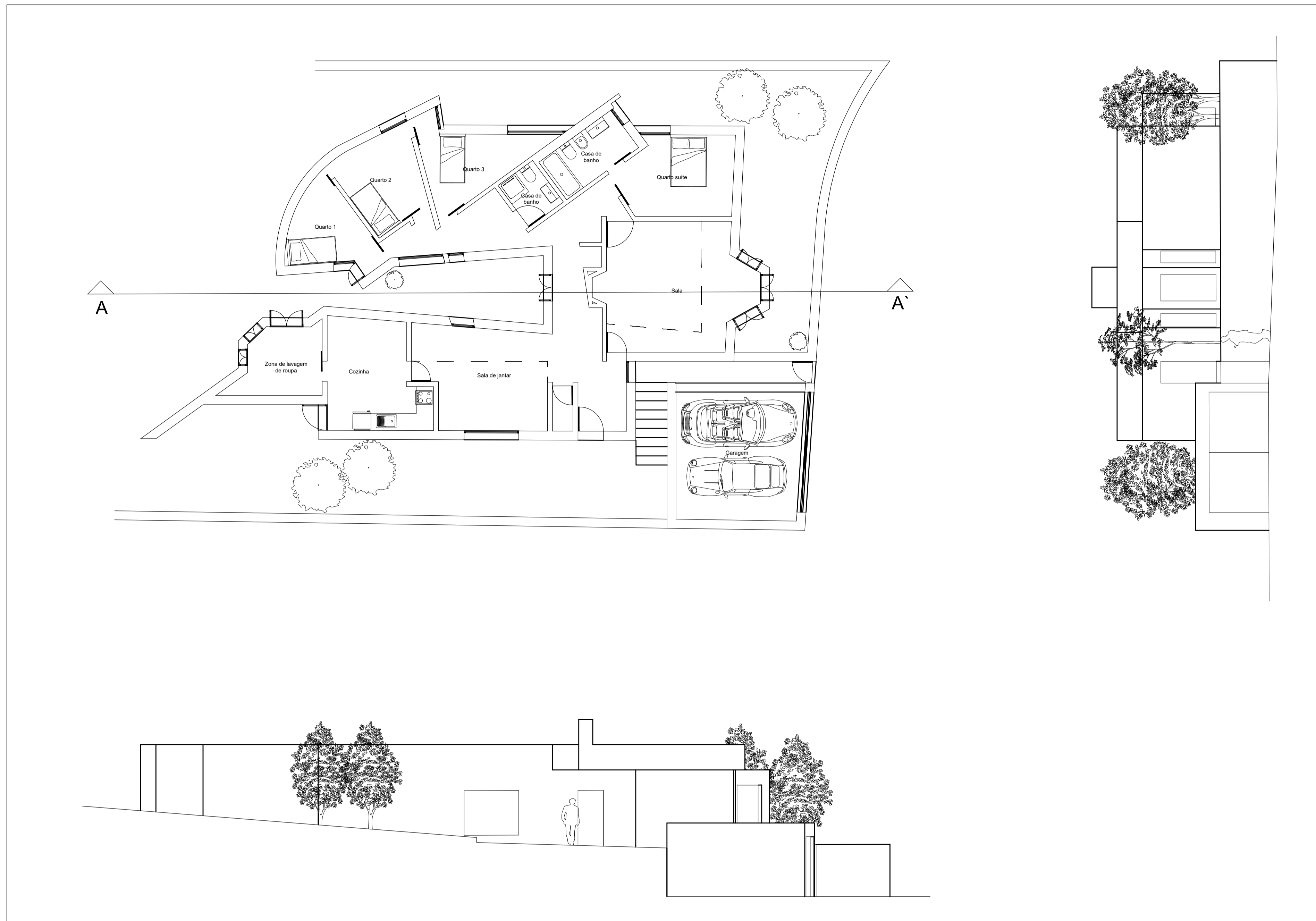
Planta e Alçados 1/100
